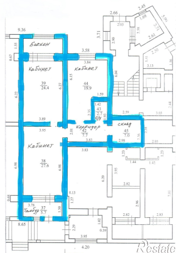
План нежилых помещений Офиса №5 по адресу: ул. Офицерская, д.4А
